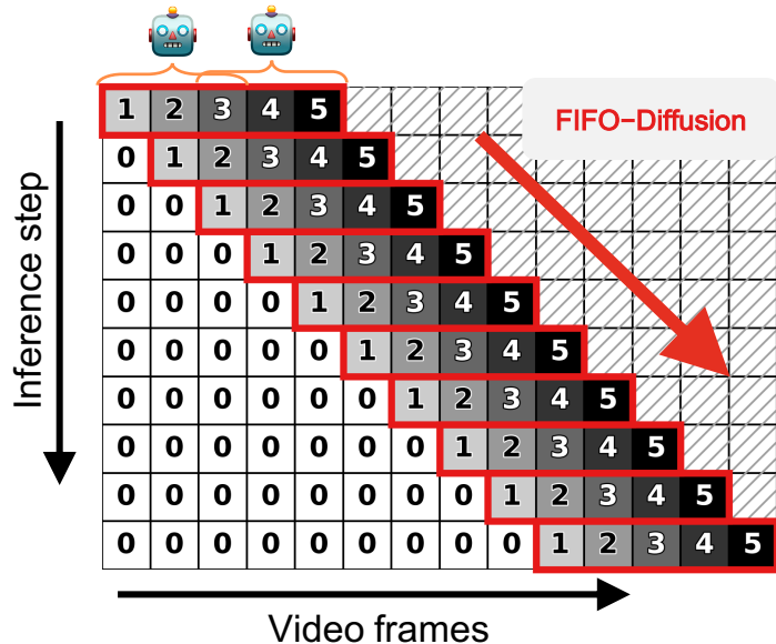
(a) FIFO-Diffusion
