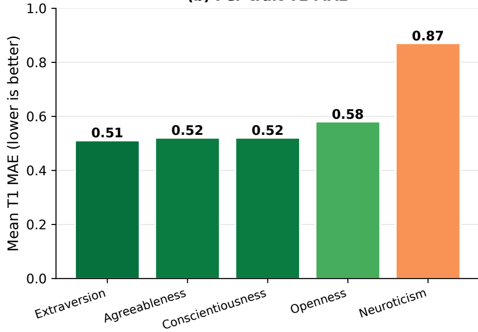
(b) Per-trait T1 MAE
