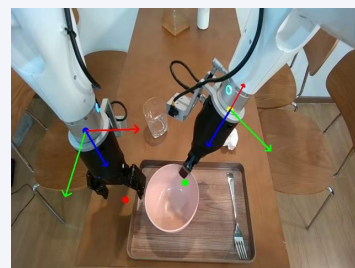
Agibot World
