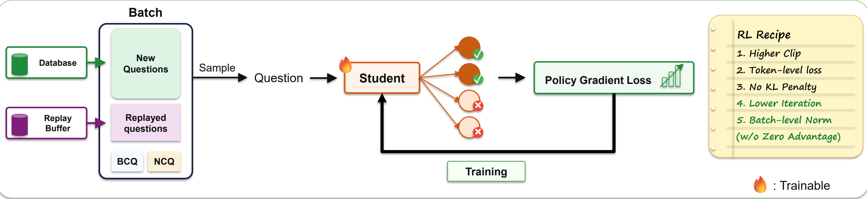
(d) Overview of ZPPO
