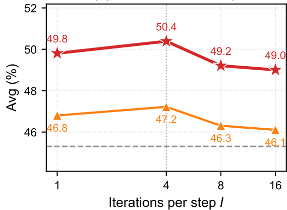
(a) 10 LLM · / sweep
