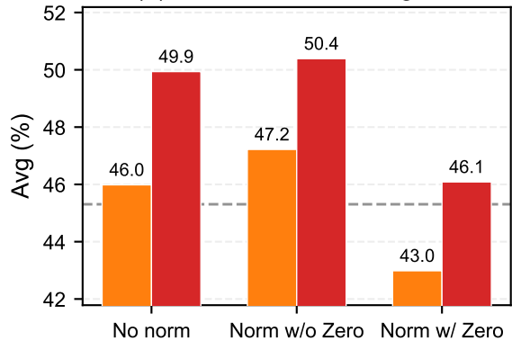
(d) 10 LLM · Norm regime
