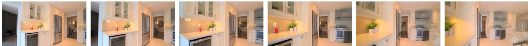
Ours
