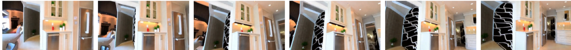
Voyager
