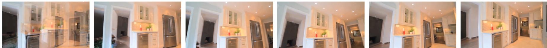
Spatia
