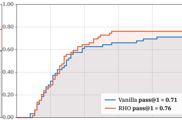
Terminal-Bench 2
