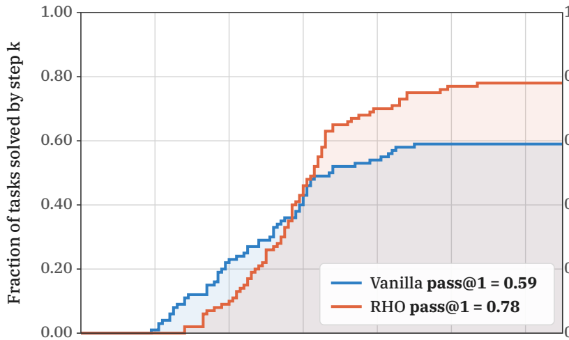
SWE-Bench Pro
