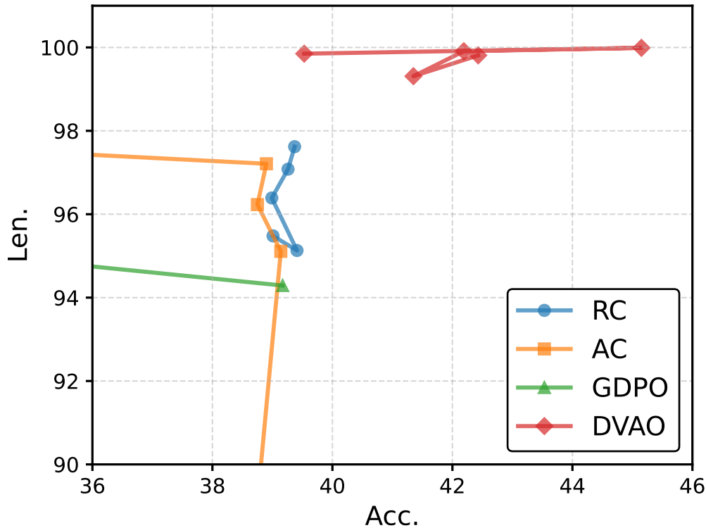
Qwen3-4B-Base
