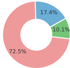
BrowseComp-zh
