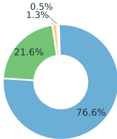
BrowseComp-zh
