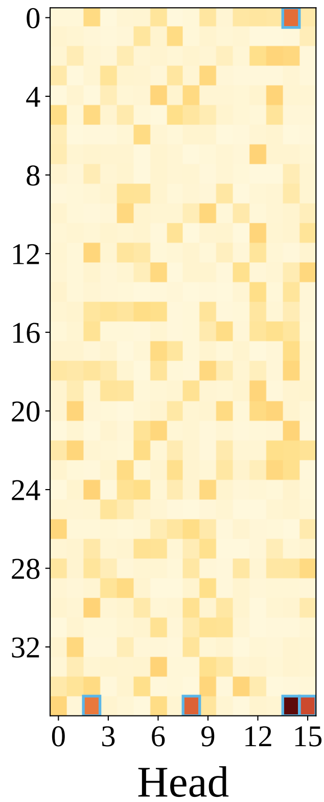
S2TT
