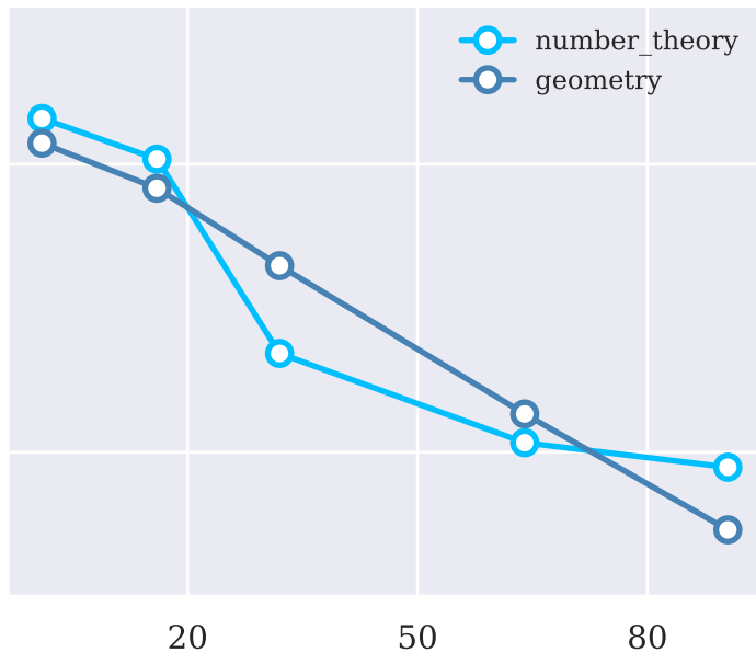
(a) Llama 3.3
