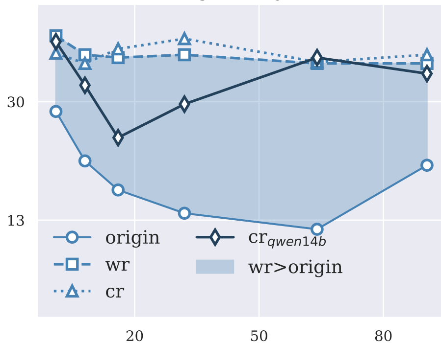
(a) Llama 3.1
