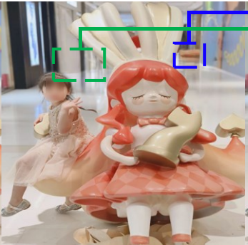
Moebius
