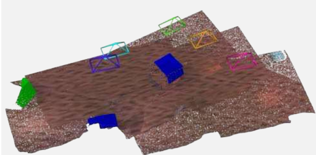
DA3
