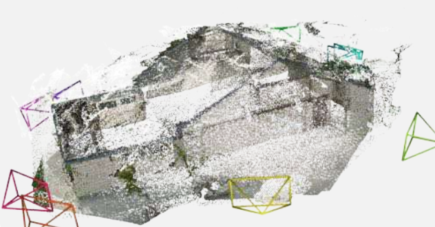
Pi3-X
