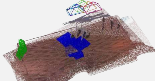
OmniVGGT
