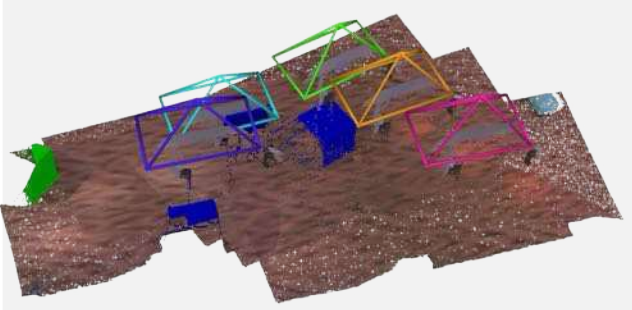
Pi3-X
