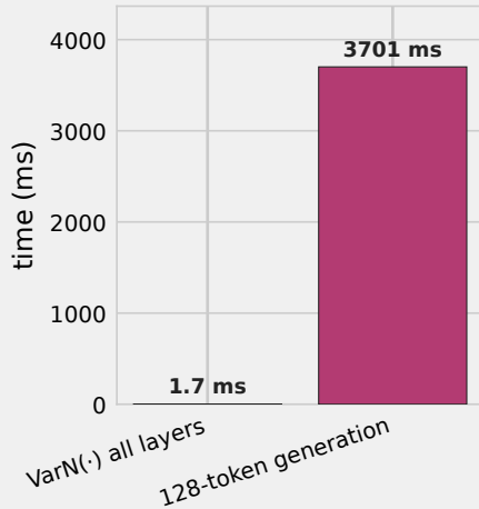
Llama-3.1-8B
