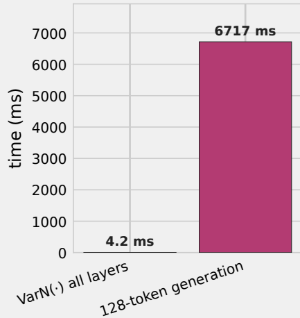
Phi-4-14B
