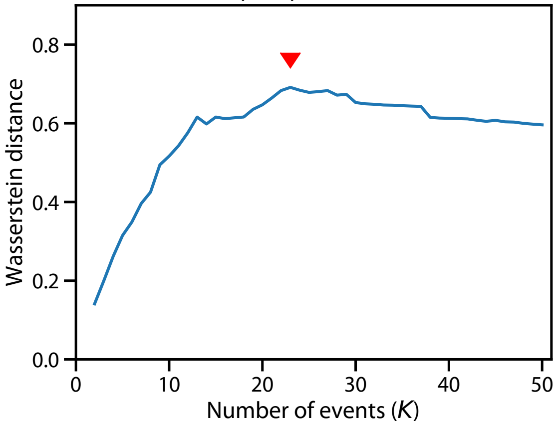
atlep1: optimal K = 23
