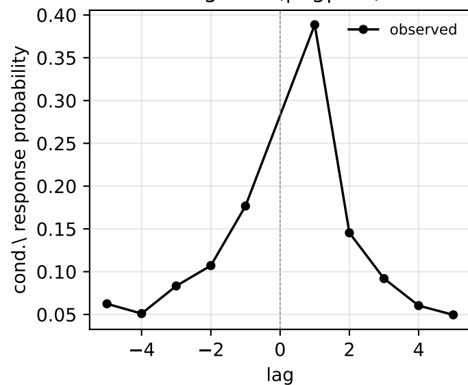
Lag-CRP ( |\text{lag}| \leq 5 )
