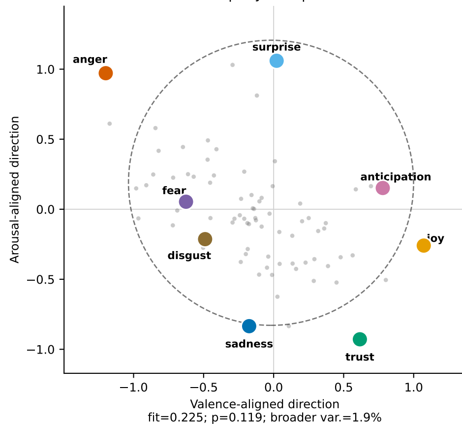
Romanian | layer 4 | PC2+PC4
