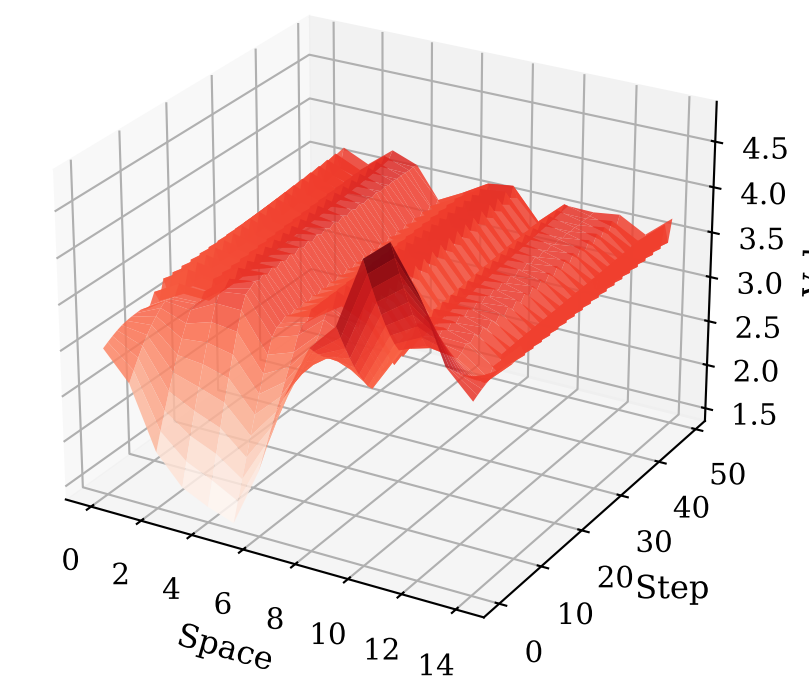
CPNODE Error
