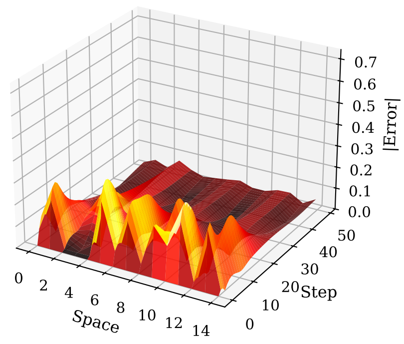
NODE-LAC Error
