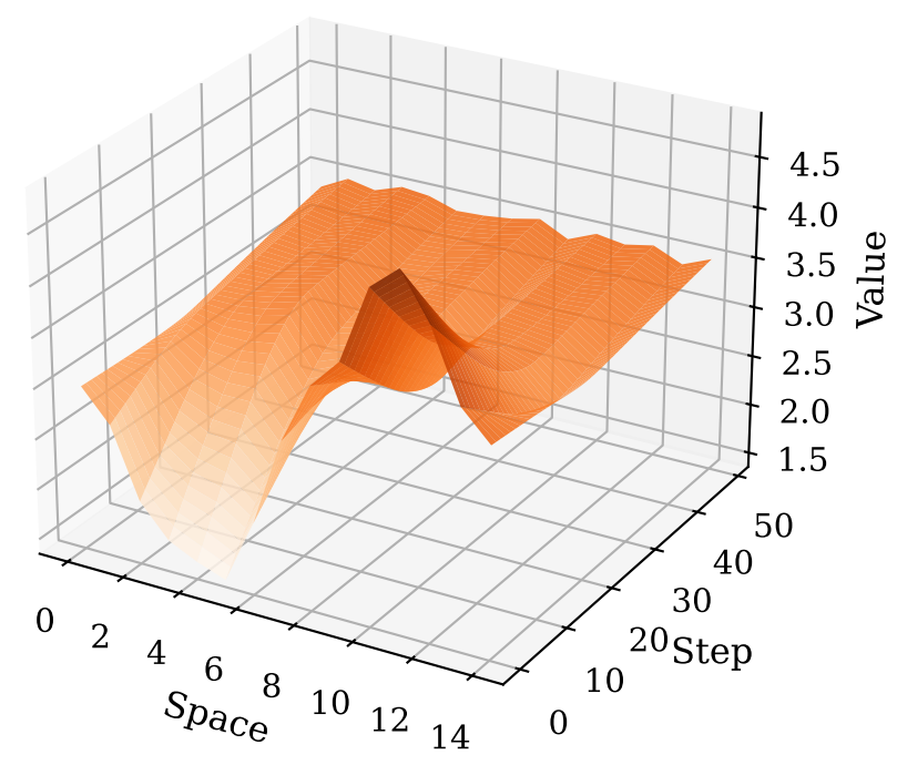
NODE Error
