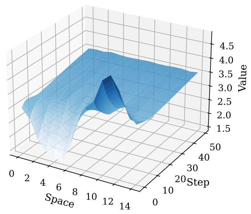
NODE-LAC Error
