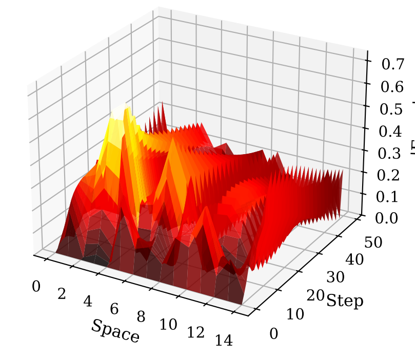
CPNODE Error
