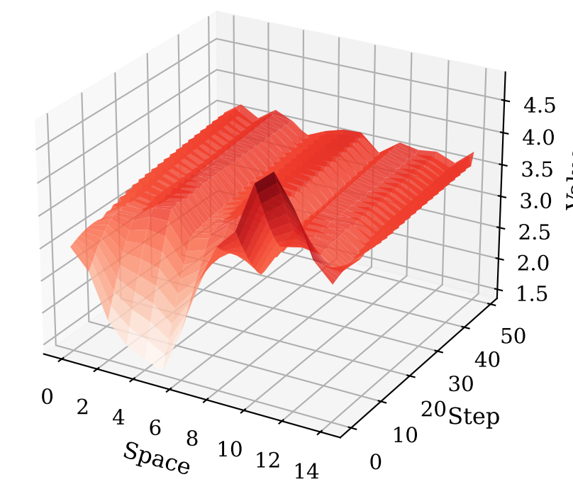
PNODE Error
