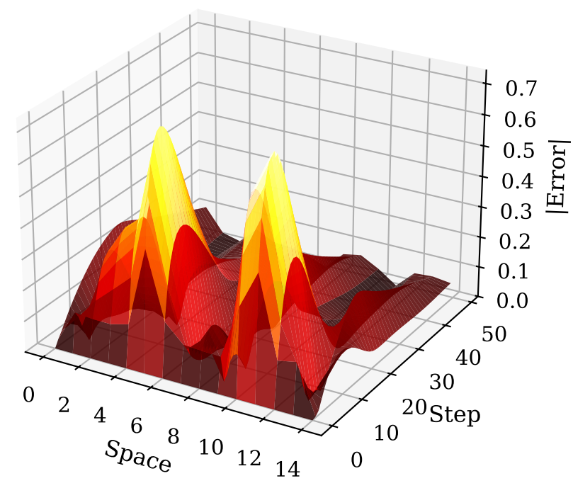
NODE Error
