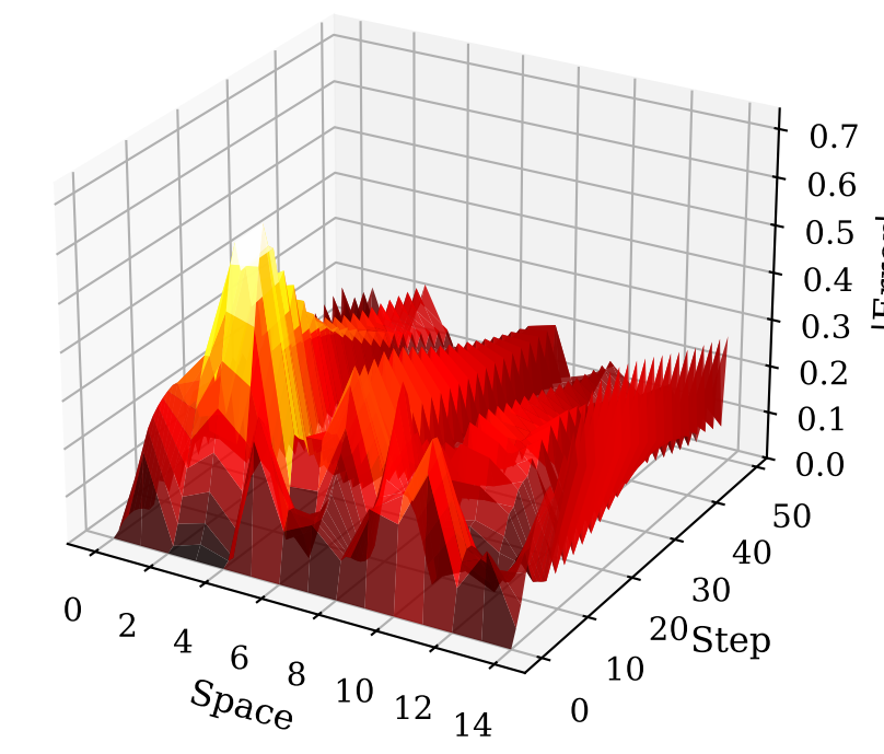
PNODE Error
