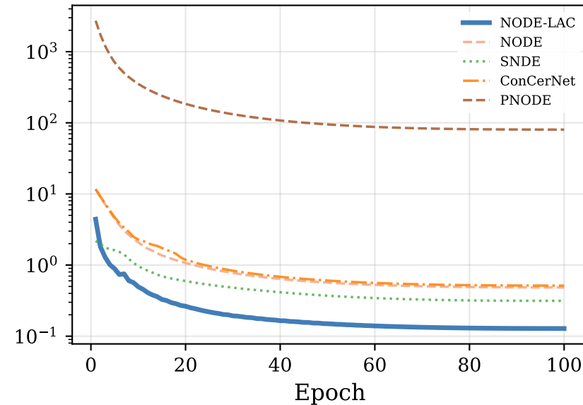
Lotka-Volterra
