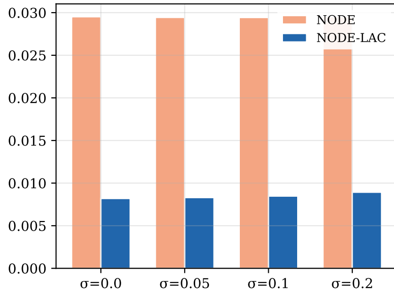
Lotka-Volterra
