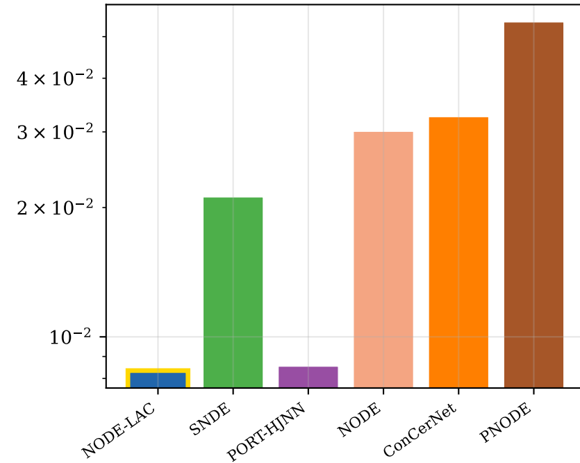
Lotka-Volterra
