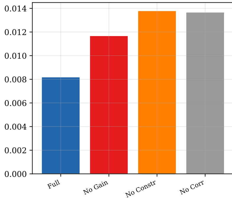
Lotka-Volterra
