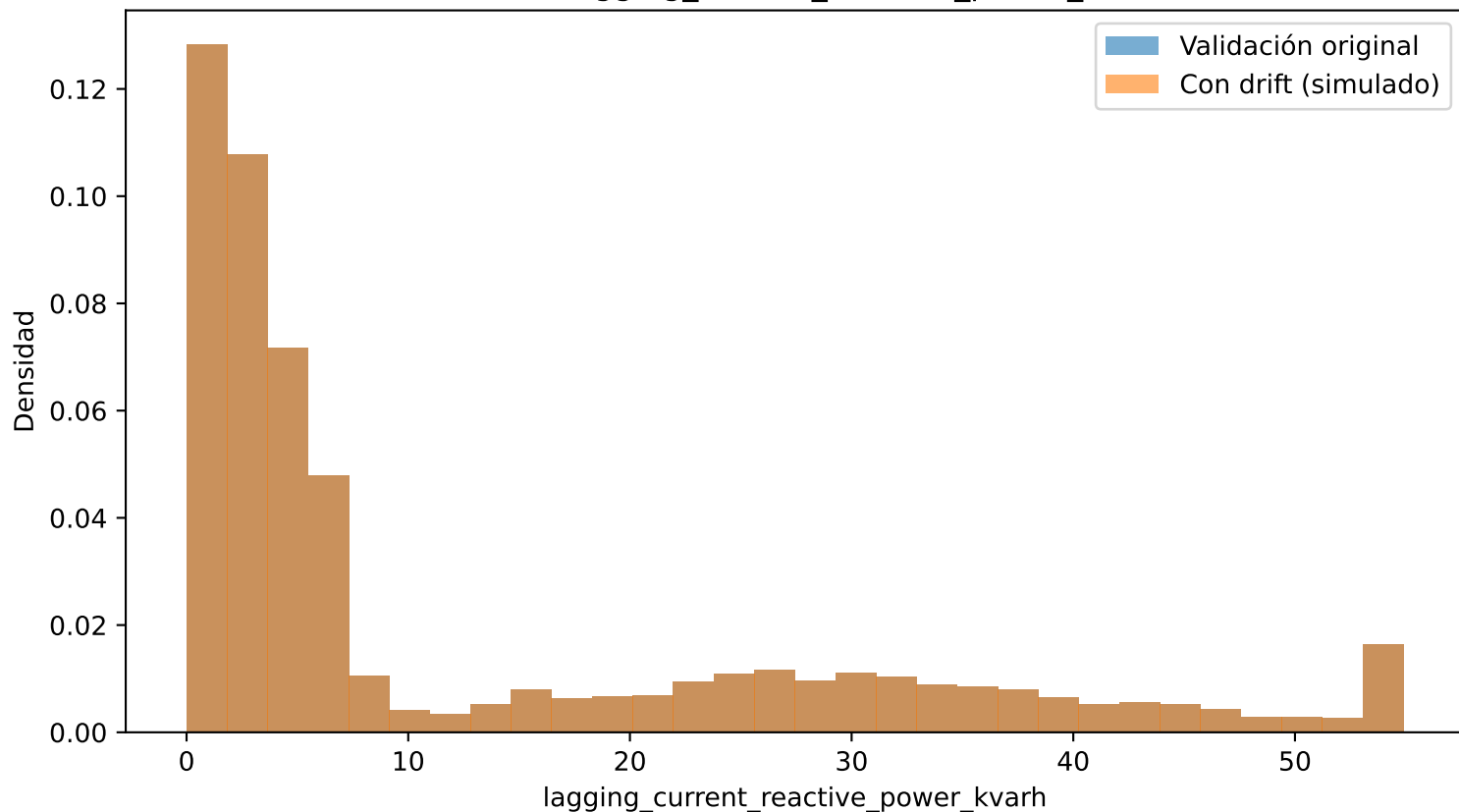
Comparación de distribuciones antes y después del drift Variable: lagging_current_reactive_power_kvarh
