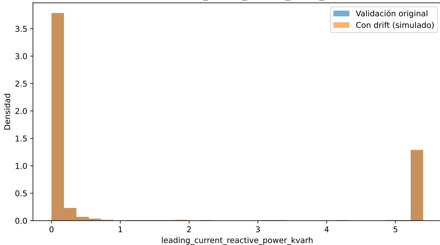
Comparación de distribuciones antes y después del drift Variable: leading_current_reactive_power_kvarh
