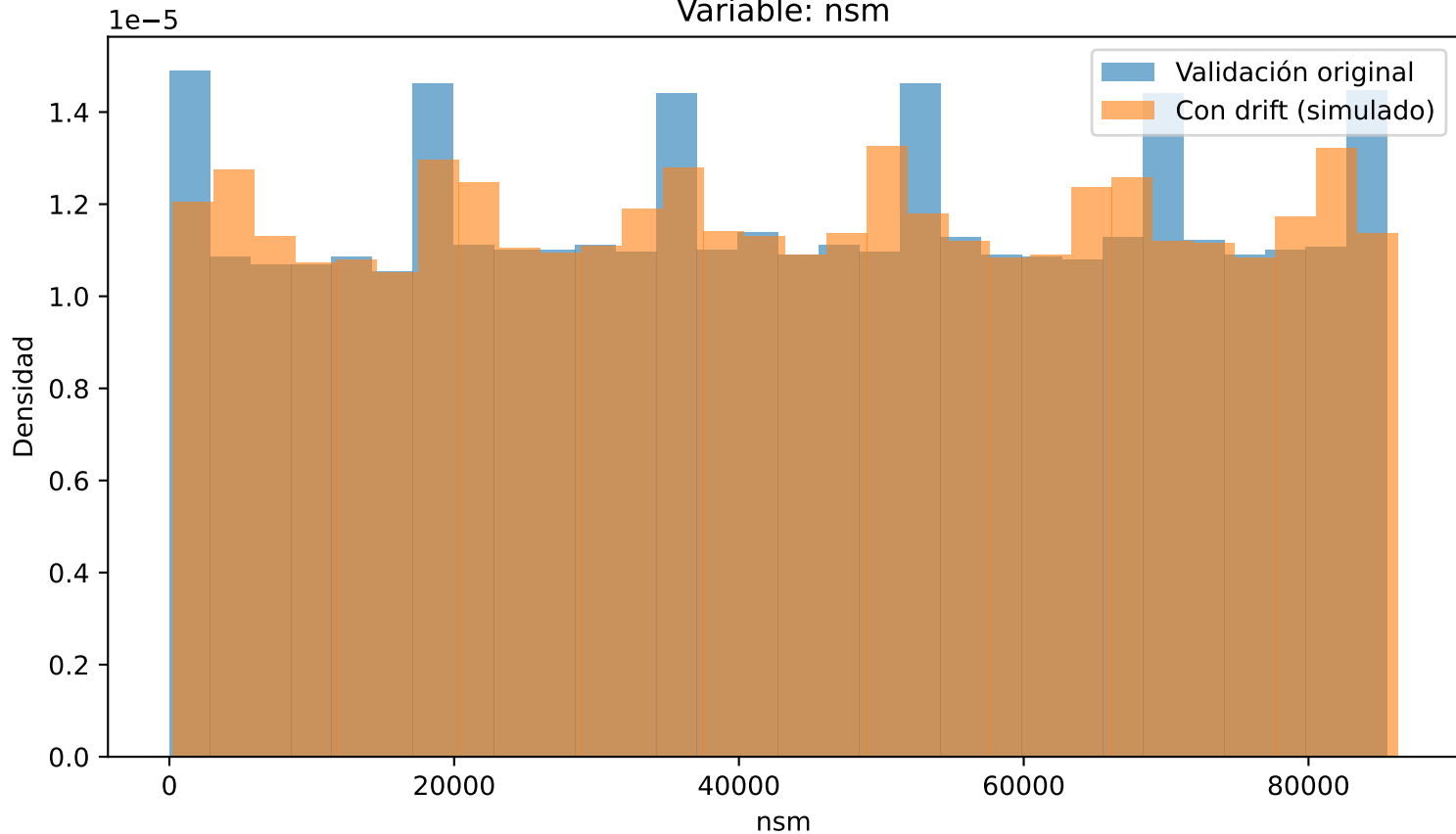
Comparación de distribuciones antes y después del drift Variable: nsm
