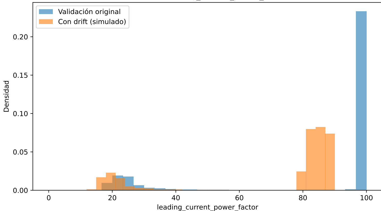
Comparación de distribuciones antes y después del drift Variable: leading_current_power_factor
