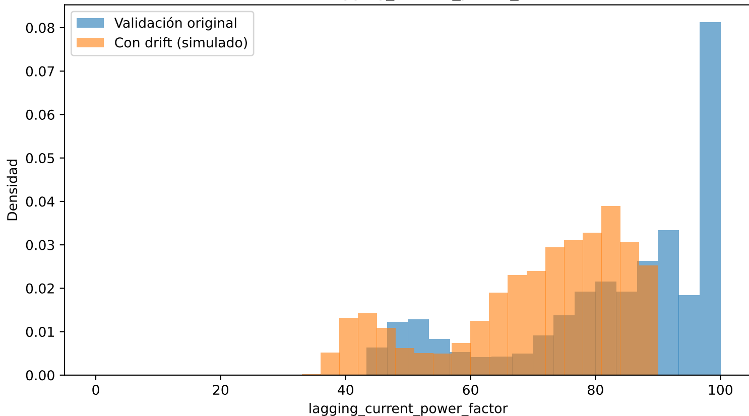
Comparación de distribuciones antes y después del drift Variable: lagging_current_power_factor
