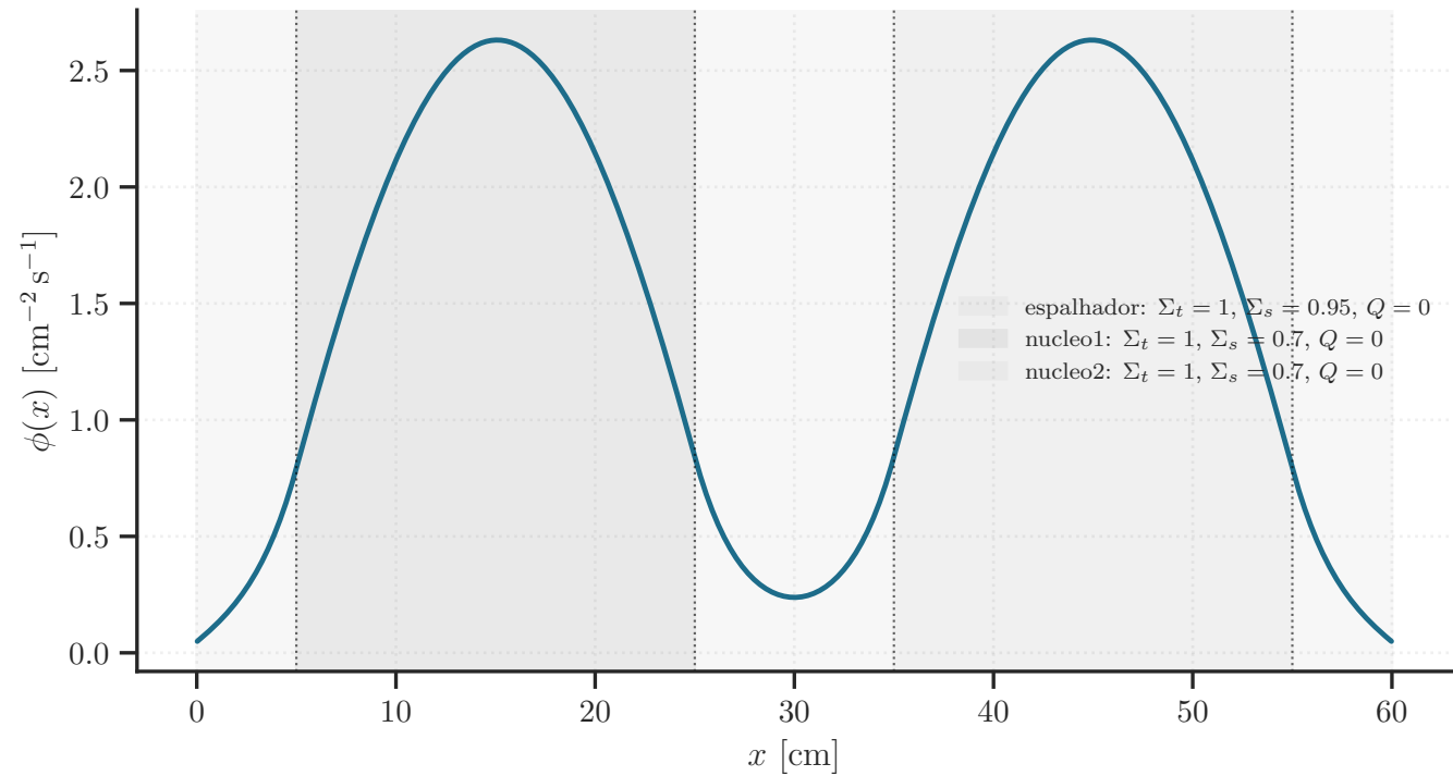
Autovalor 1D — dois núcleos fracamente acoplados (Wielandt) ( k_{\text{eff}} = 1.277647 )
