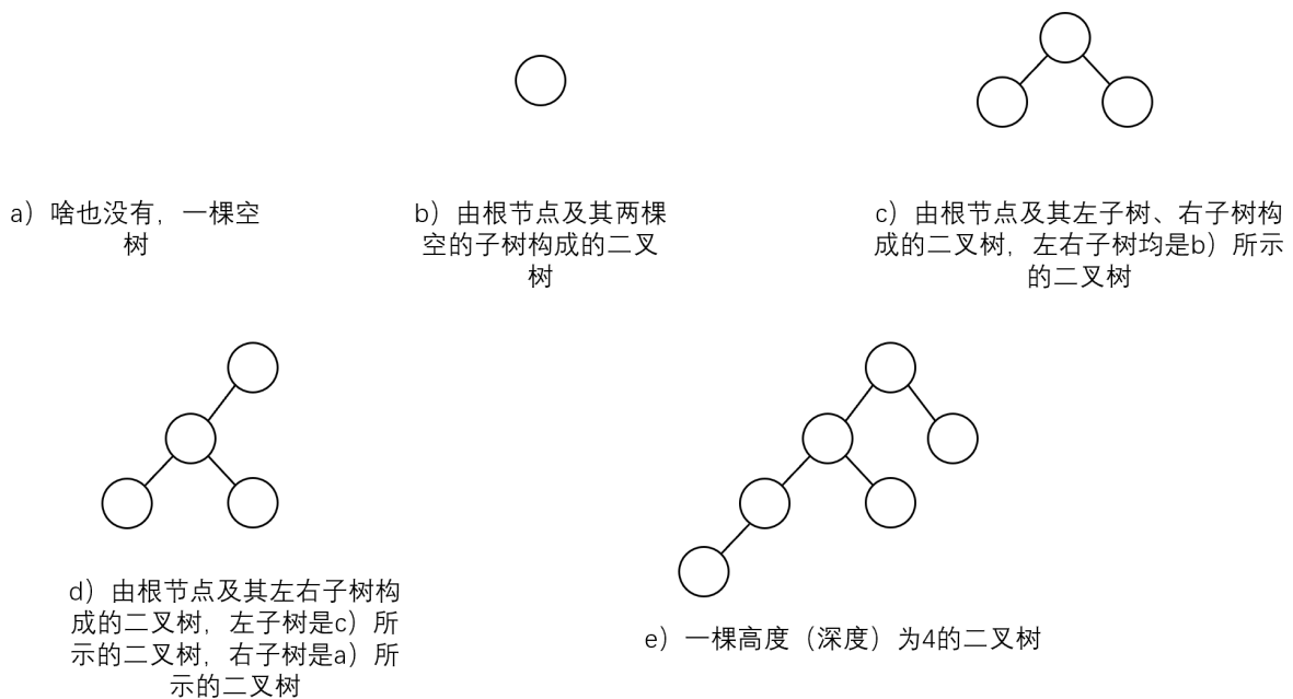
图 4.4 几棵不同的二叉树
