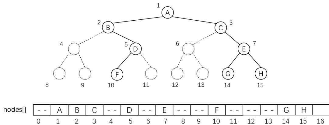
图 4.6 用数组存储二叉树
