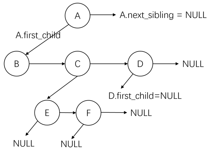
图 4.2 树的孩子-兄弟表示法
