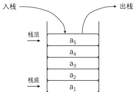
图 3.2 栈的示意图
