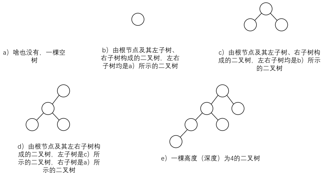
图 4.4 几棵不同的二叉树
