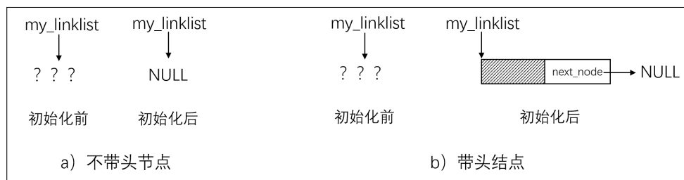
图 2.5 链表初始化前后示意
