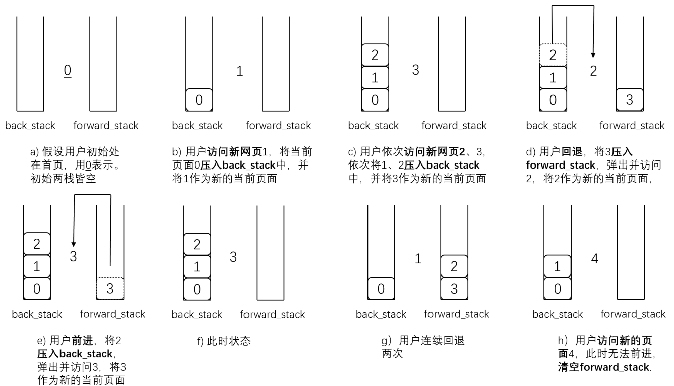
图 3.6 使用两个栈实现浏览器前进后退
