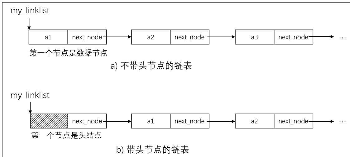
图 2.6 带头节点与不带头节点的链表
