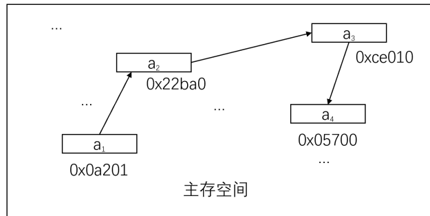
图 2.3 链式存储的线性表
