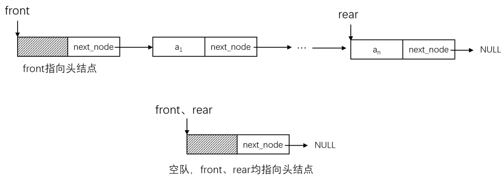
图 3.7 带头结点的链式队列示意图
