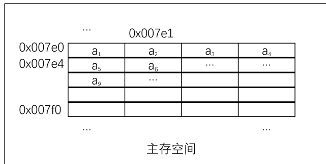
图 2.1 顺序存储的线性表
