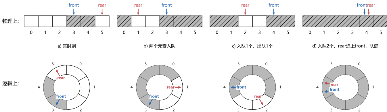
图 3.10 循环队列示意图
