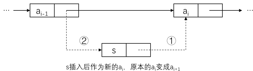
图 2.7 链表的插入过程示意
