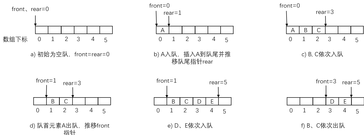
图 3.9 在顺序表上实现队列
