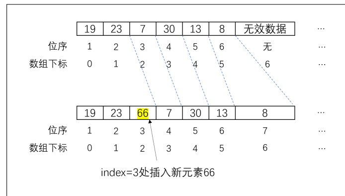
图 2.4 顺序表的插入操作
