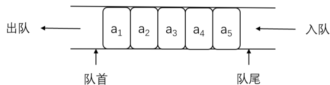
图 3.3 队列示意图
