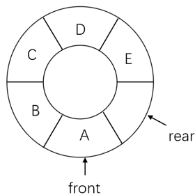
图 3.11 队满示意图
