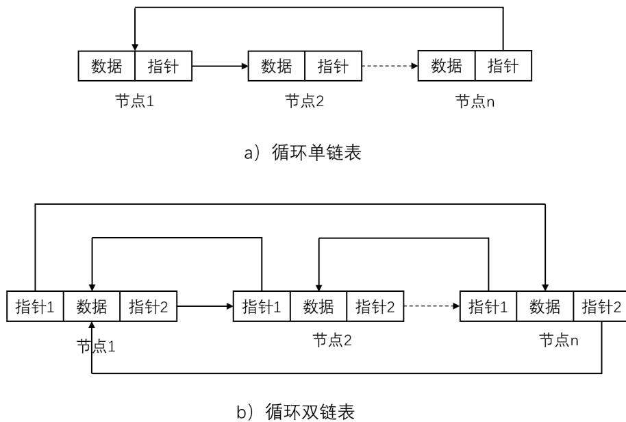
图 2.10 循环链表示意图
