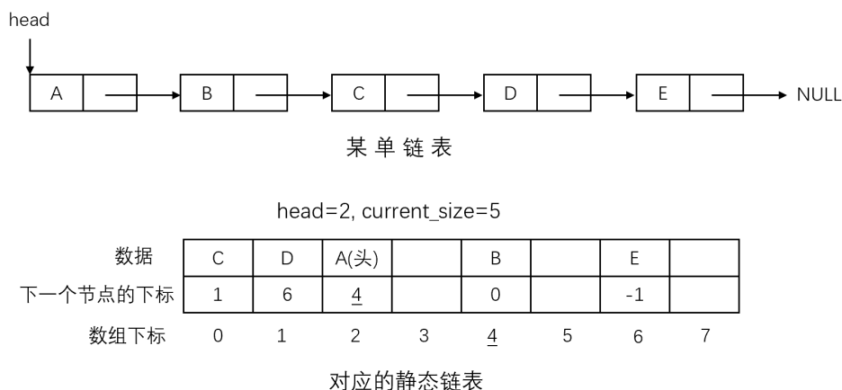
图 2.11 静态链表示意图
