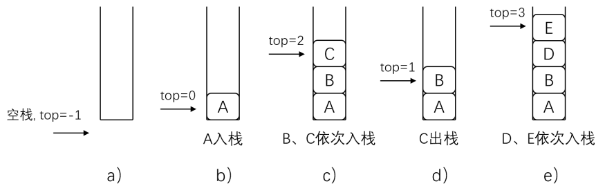
图 3.4 顺序栈实现示意图
