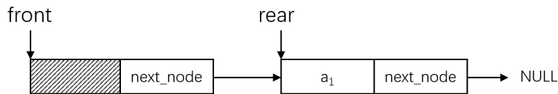
图 3.8 仅有一个数据节点的队列
