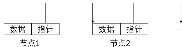
图 2.2 链表的节点
