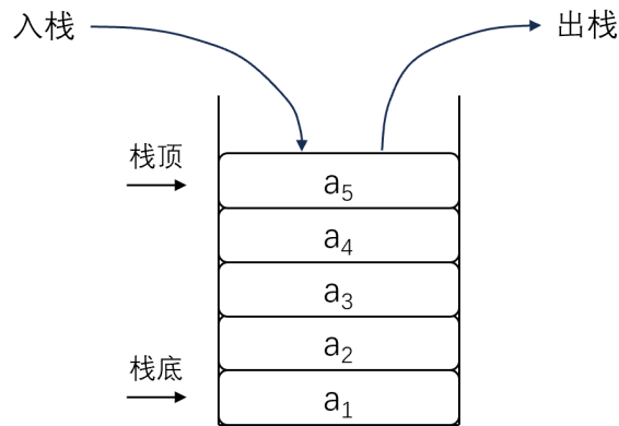
图 3.2 栈的示意图
