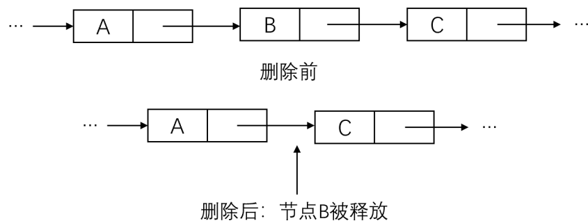
图 2.8 链表的删除过程示意
