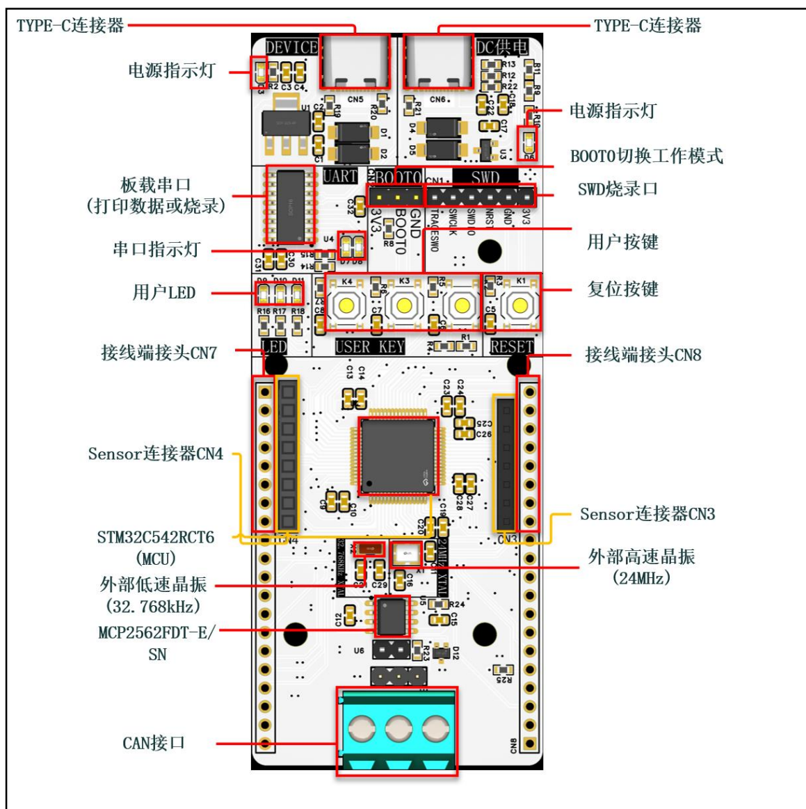
图 1 STM32C542R & SENSOR 开发板（正面）
