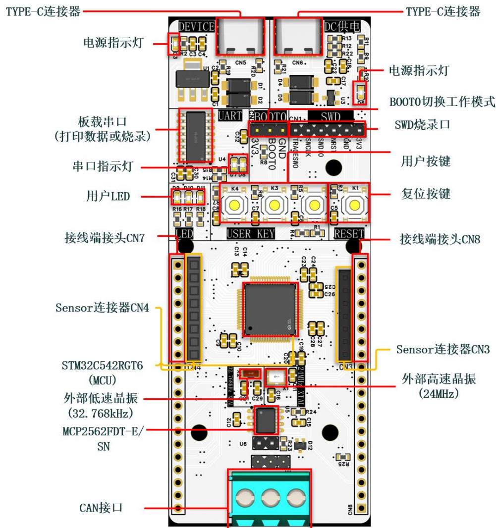
图 1 STM32C542R & SENSOR 开发板 (正面)
