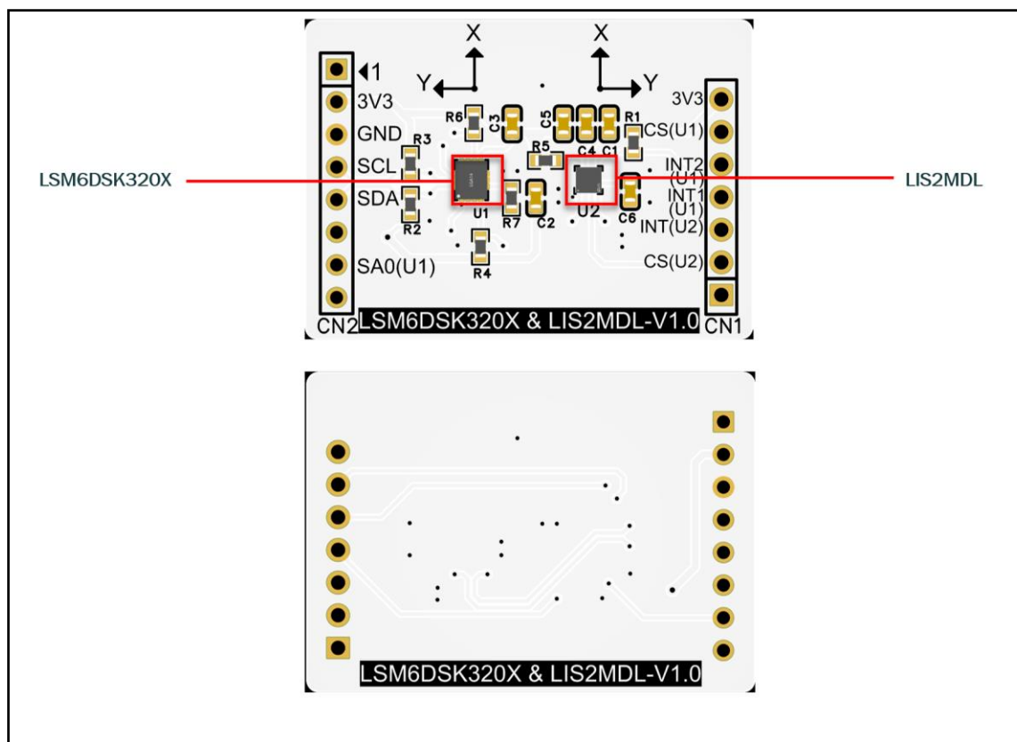
图 1 LSM6DSK320X & LIS2MDL 评估套件
