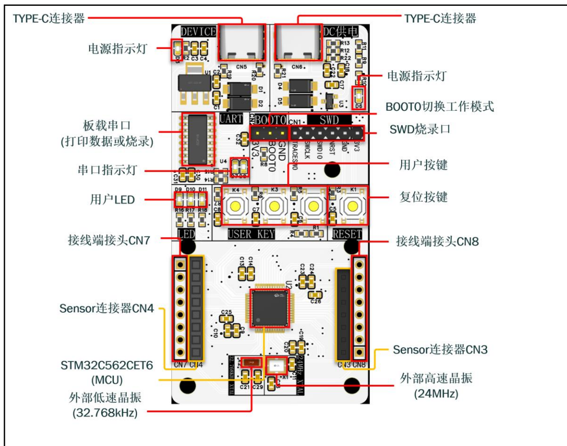
图 1 STM32C562 & SENSOR 开发板 (正面)
