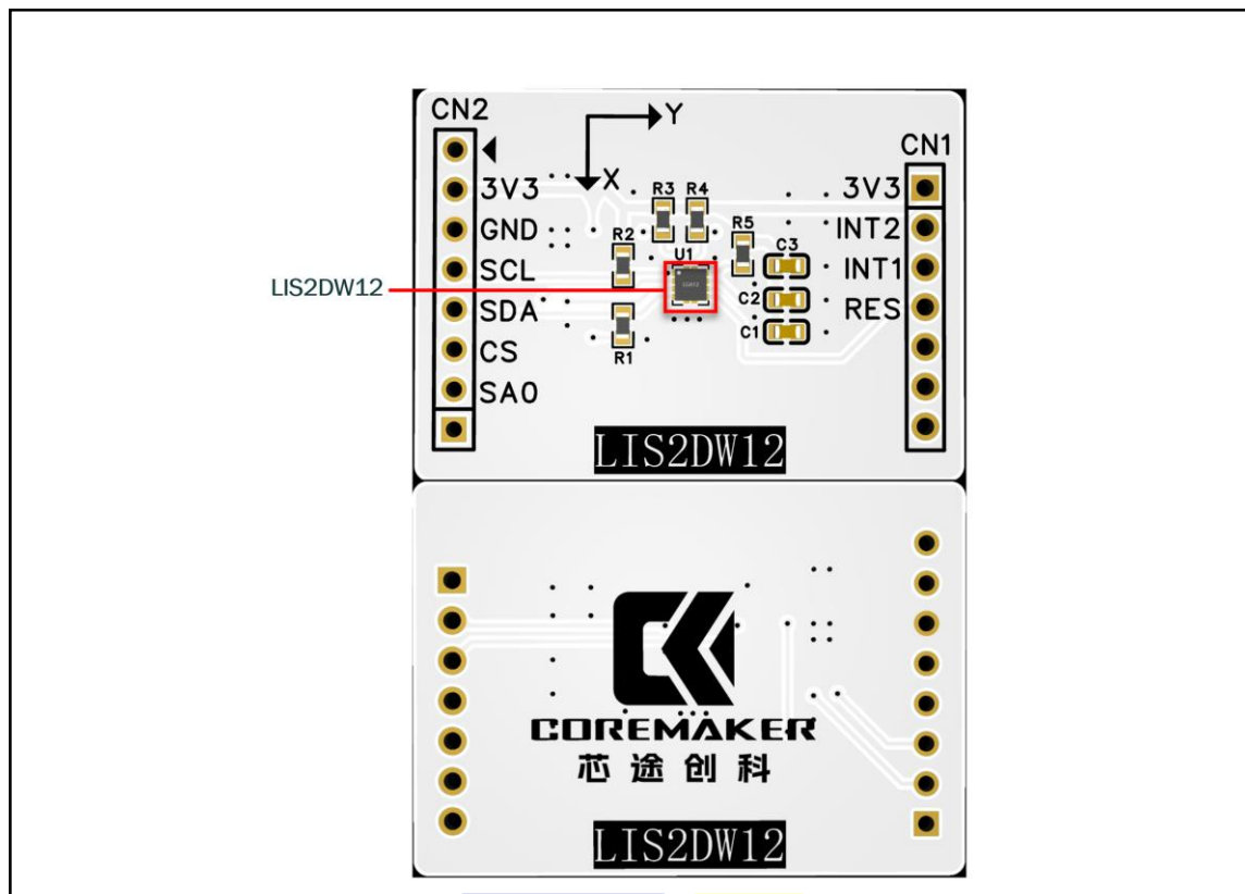
图 1 LIS2DW12 评估套件
