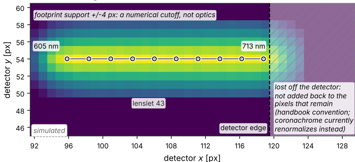
(c) detector edge
