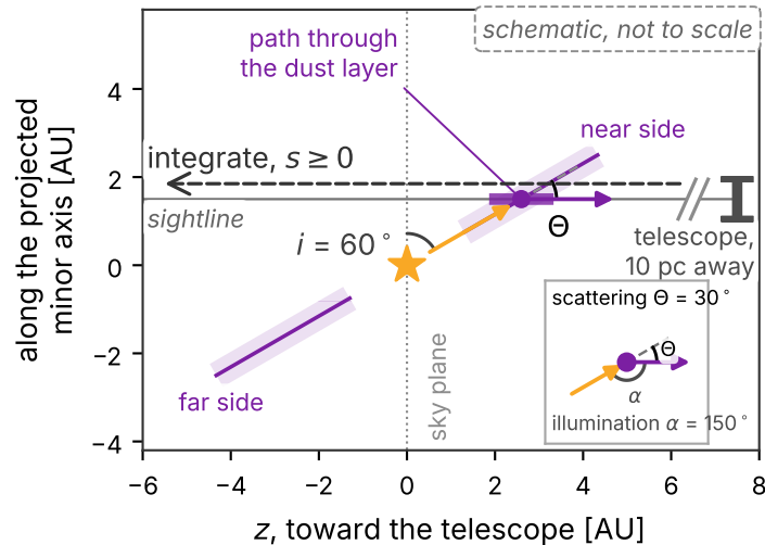
(b) side on: inclination i
