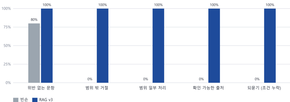
빈손 대비 최종(v3) · 지킨 비율 (%)
