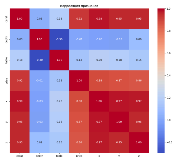
Рис. 2: Матрица корреляций
