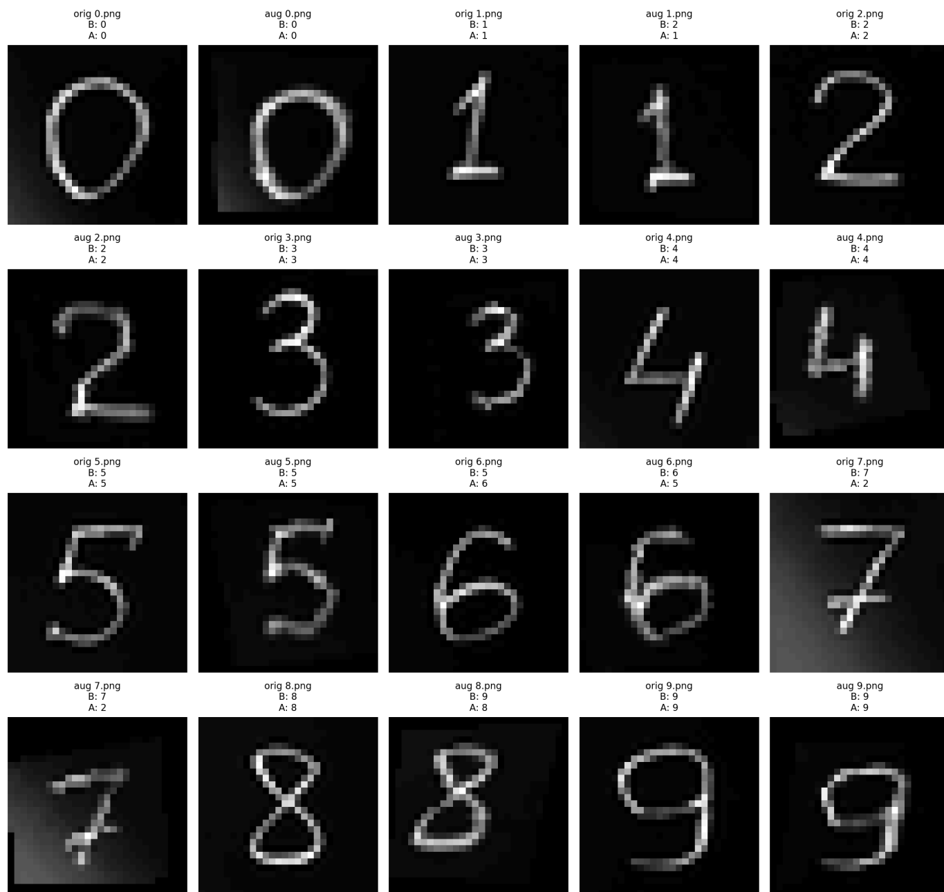
Рис. 15: Сравнение предсказаний baseline CNN и CNN с аугментацией на обычных и аугментированных собственных изображениях
