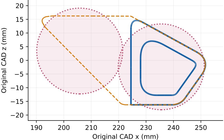
Longitudinal section: CAD y = 1 mm
