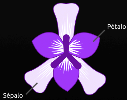
Iris-Versicolor
