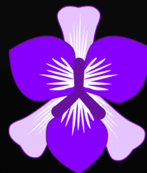
Iris-Virginica
