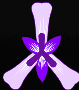
Iris-Setosa
