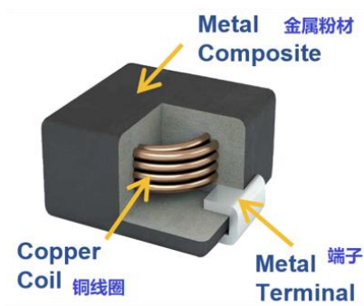
产品结构图 Product structure diagram
