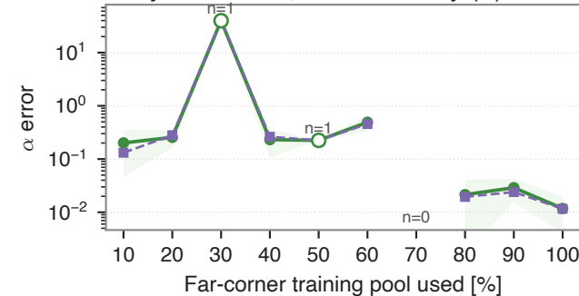
Ansys validation, anharmonicity ( \alpha )
