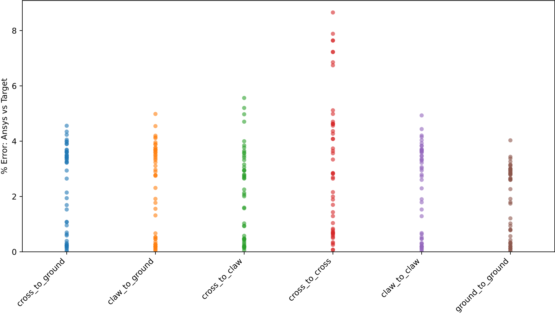
Per-Capacitance Error: Ansys vs Target Capacitance (all sigmas)
