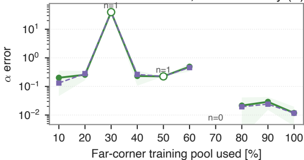
EM simulator validation, anharmonicity ( \alpha )
