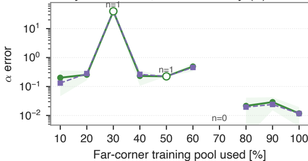
Ansys validation, anharmonicity ( \alpha )
