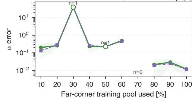
EM simulator validation, anharmonicity ( \alpha )
