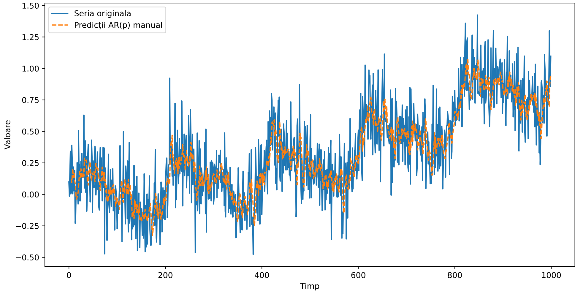
Seria originală vs Predictii AR
