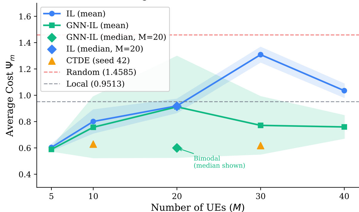
Scaling Performance: IL vs GNN-IL
