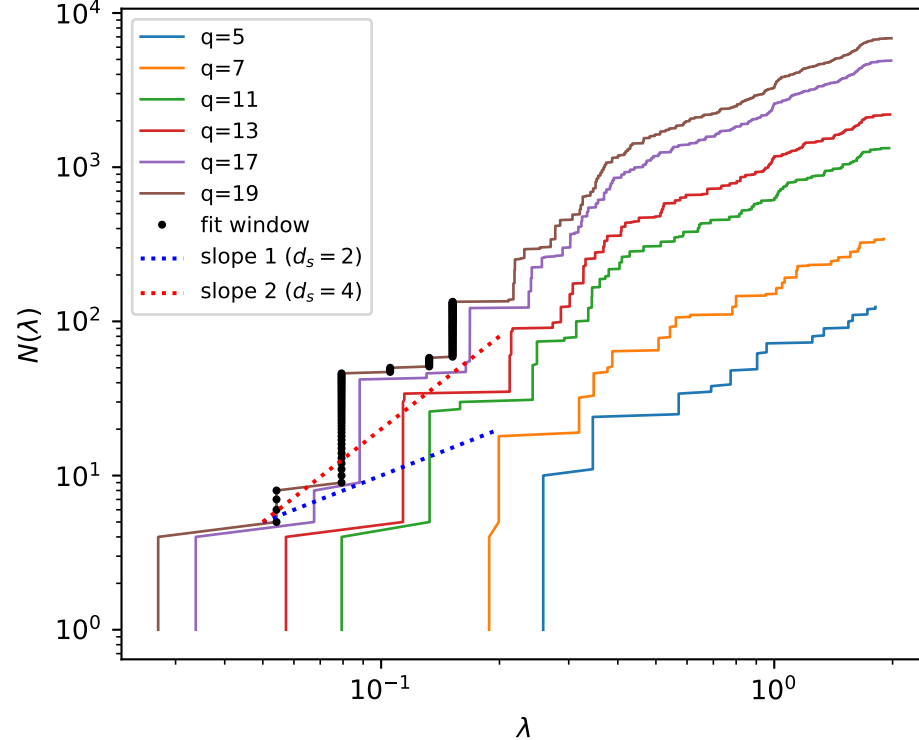
Edge integrated DOS
